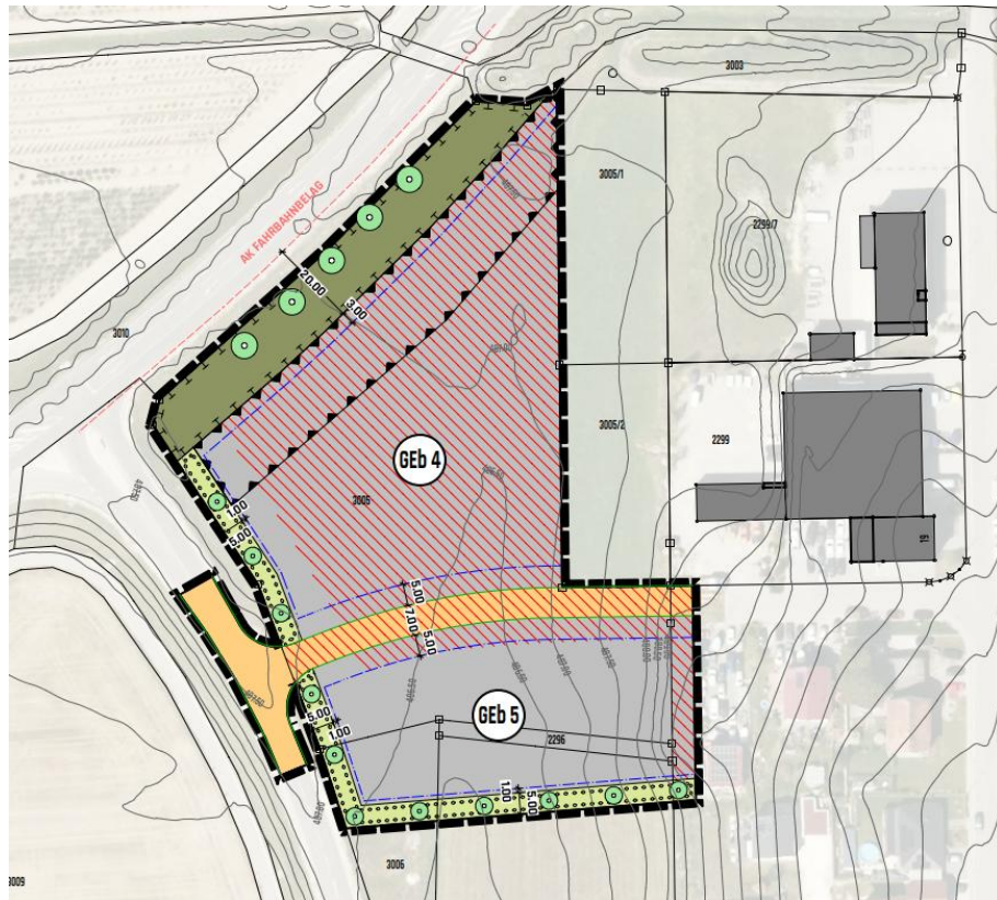
Planauszug Bebauungsplan unmaßstäblich
